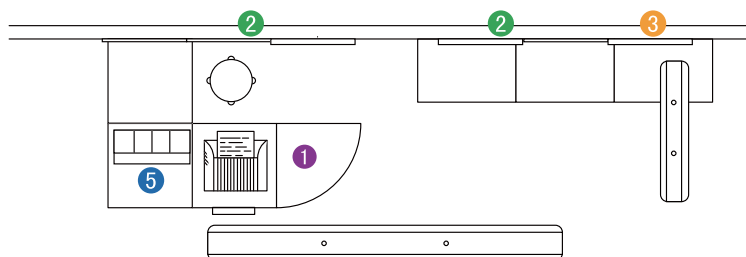
背靠单面墙店中店布局图 占地面积约4.7m 2
