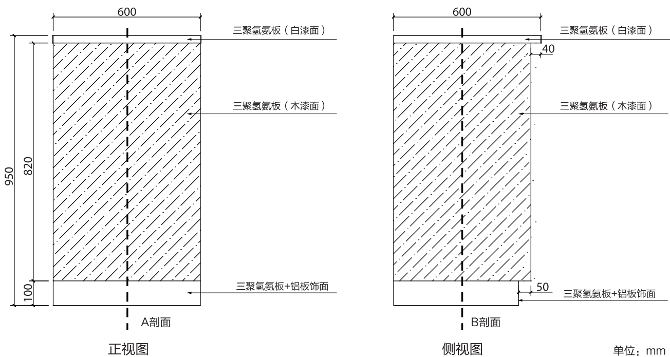
■ 销售柜台结构图
