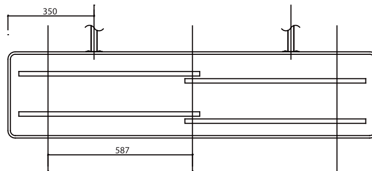
灯管规格1500*350，制作工艺同2000*350规格，灯具和吊杆分布如图 灯管：24WT4灯管
