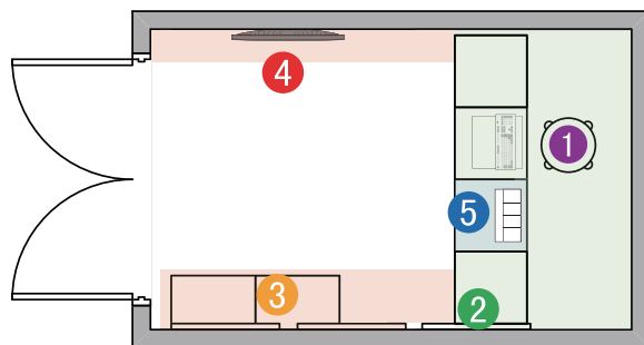
细长形店面布局 约10m 2 (4m x 2.5m)
