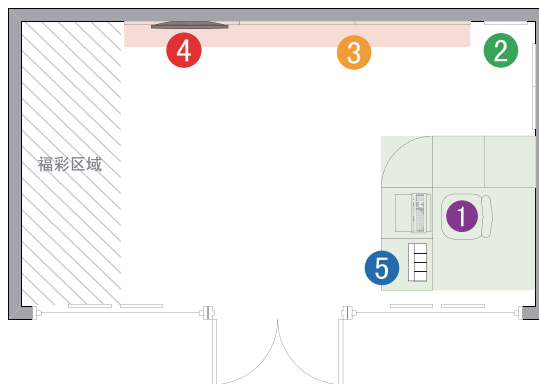
扁宽形店面布局 约20m 2 (5.5m x 3.6m)
